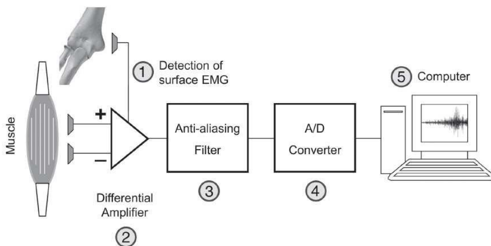
ภาพที่ 14 ส่วนประกอบพื้นฐานของระบบตรวจวัดสัญญาณ EMG (Surface EMG acquisition system)
